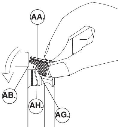
Abb. 9 Einsetzen und Entfernen der Schauglaskappe
