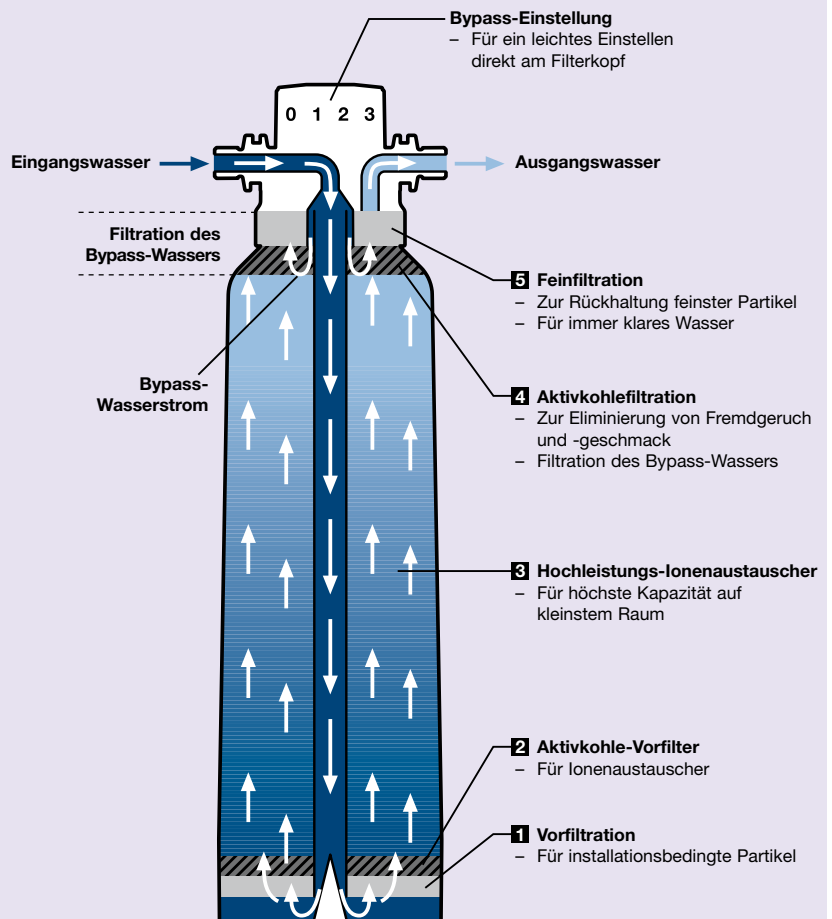
Aufbau einer BWT bestprotect Filterkerze mit 5-fach-Filtration
