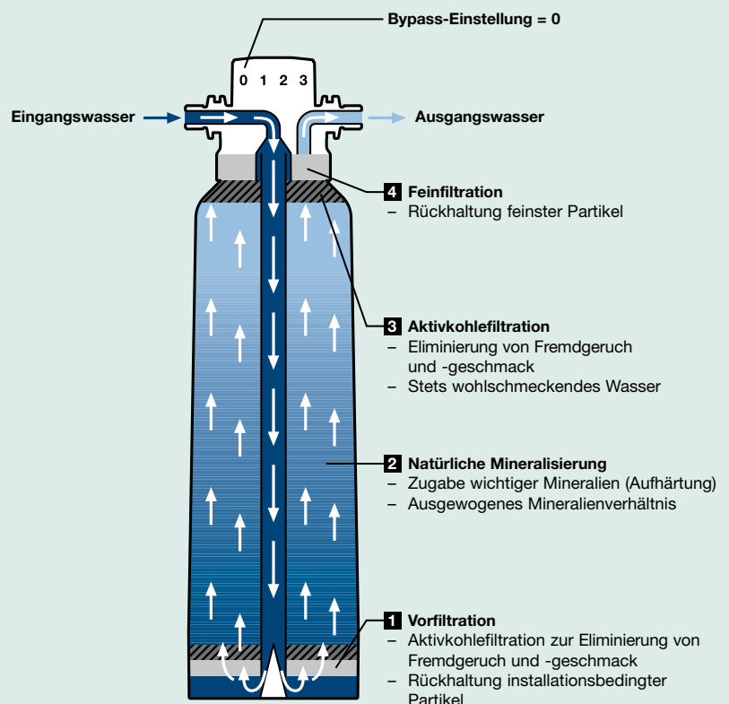
Aufbau einer BWT bestmin Filterkerze
