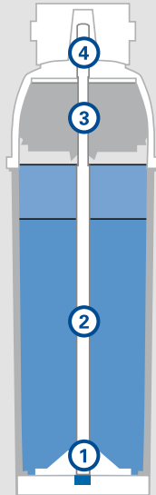
Die gezeigte Illustration dient nur zur Ansicht und Erläuterung der Filtertechnologie. Sie ist nicht maßstabstreu und zeigt beispielhaft den Querschnitt der Filtergröße C150.
